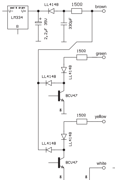
Výstupový diagram OD 07-24S a OD 07-24V
